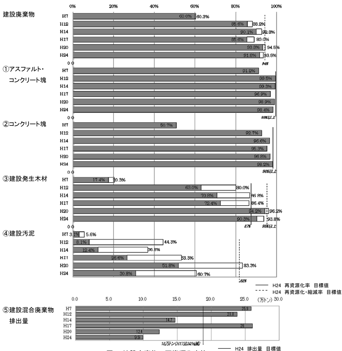
図5. 建設廃棄物の再資源化率等
