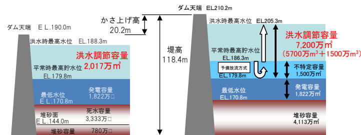
【丸山ダム】
