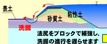
越水による堤防裏法尻の洗掘イメージ
